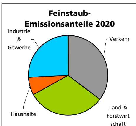
Abb. 22 Anteile der Feinstaub-Emissionen im Jahre 2020 Quelle: 'Weiterentwicklung des Luftreinhaltekonzeptes' Schriftenreihe Umwelt Nr. 379, BUWAL, 2005 [44]
