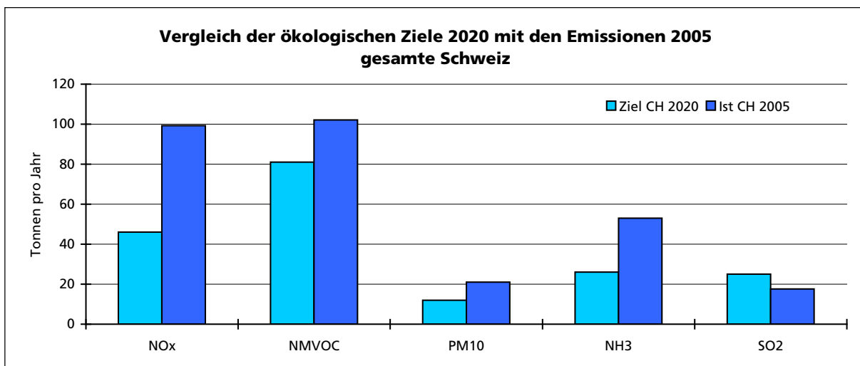
Abb. 26 Quantifizierung der ökologischen Ziele für das Jahr 2020 [44] und der im Jahre 2005 emittierten Schadstoffmengen [91] für die gesamte Schweiz. Die Differenzen der beiden Säulen ergeben die jeweiligen Ziellücken (gesamte Schweiz).
