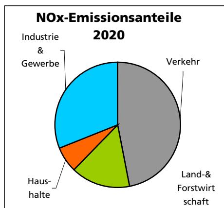
Abb. 16 Anteile der Stickoxid-Emissionen im Jahre 2020 Quelle: 'Weiterentwicklung des Luftreinhaltekonzeptes' Schriftenreihe Umwelt Nr. 379, BUWAL, 2005 [44]
