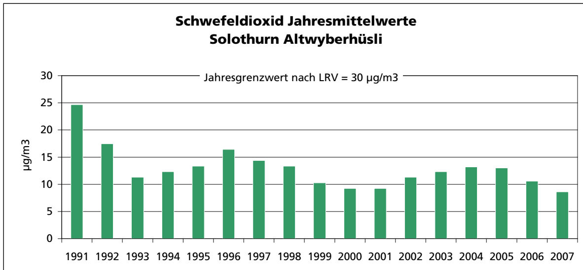
Abb. 3 Die Schwefeldioxidbelastung wird lediglich noch bei der Messstation Altwyberhüsli in Solothurn gemessen. Die Jahresmittelwerte zwischen 1991 und 2007 liegen alle unter dem Immissionsgrenzwert.
