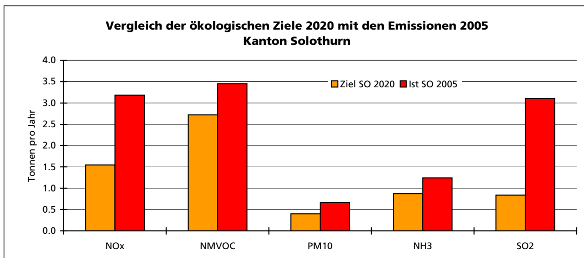
Abb. 27 Quantifizierung der ökologischen Ziele für das Jahr 2020 [44] (top-down) und der im Jahre 2005 emittierten Schadstoffmengen [97] für den Kanton Solothurn.
