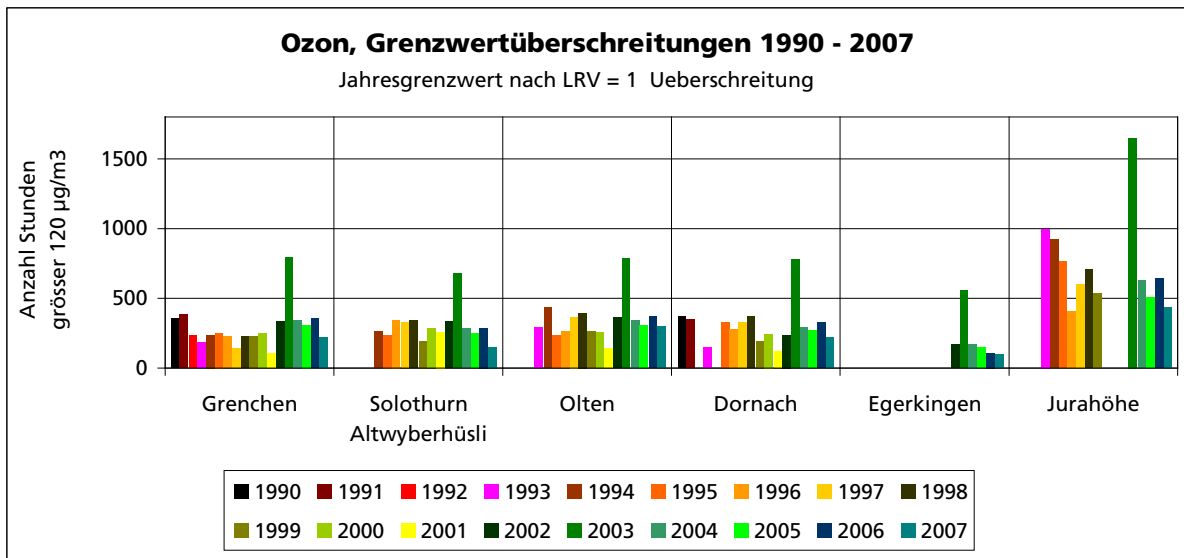
Abb. 4 Ozonbelastung im Kanton Solothurn. Dargestellt sind die Anzahl der jährlichen Überschreitungen des Stundenmittelwertes von 120 µg/m³. Nach LRV ist eine Überschreitung pro Jahr zulässig.
