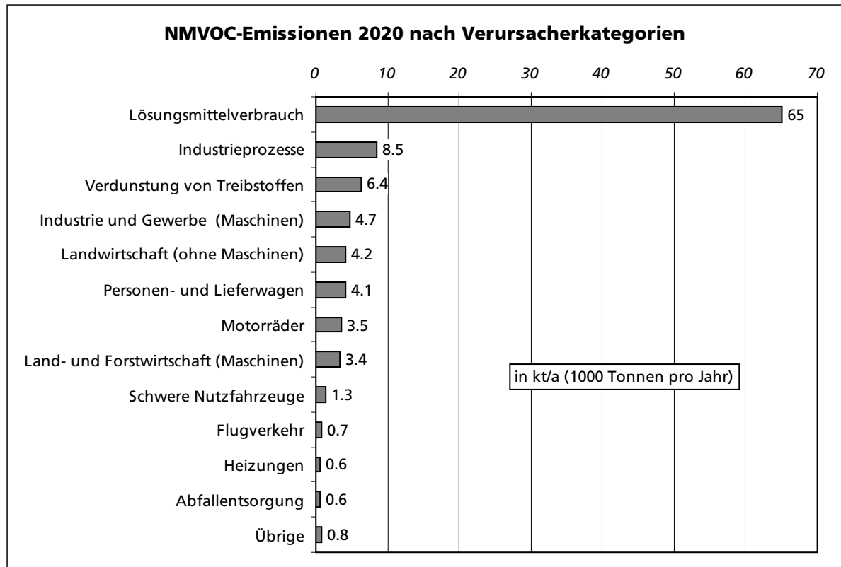
Abb. 18 NM VOC-Emissionen 2020 nach Verursacherkategorien. Die Darstellung zeigt, dass der Lösungsmittelverbrauch auch in Zukunft der Hauptverursacher für die Emissionen leichtflüchtiger organischer Verbindungen sein wird. Rund 70 Prozent der NM VOC-Emissionen entstehen durch den Einsatz dieser Stoffe in Industrie, Gewerbe und Haushalten, rund 23'000 Tonnen pro Jahr allein durch Farbanwendungen, was rund 22 Prozent der Gesamtemission entspricht. Quelle: 'Weiterentwicklung des Luftreinhaltekonzeptes' Schriftenreihe Umwelt Nr. 379, BUWAL, 2005 [44]
