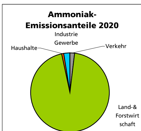
Abb. 25 Anteile der Ammoniak-Emissionen im Jahre 2020 Quelle: 'Weiterentwicklung des Luftreinhaltekonzeptes' Schriftenreihe Umwelt Nr. 379, BUWAL, 2005 [44]
