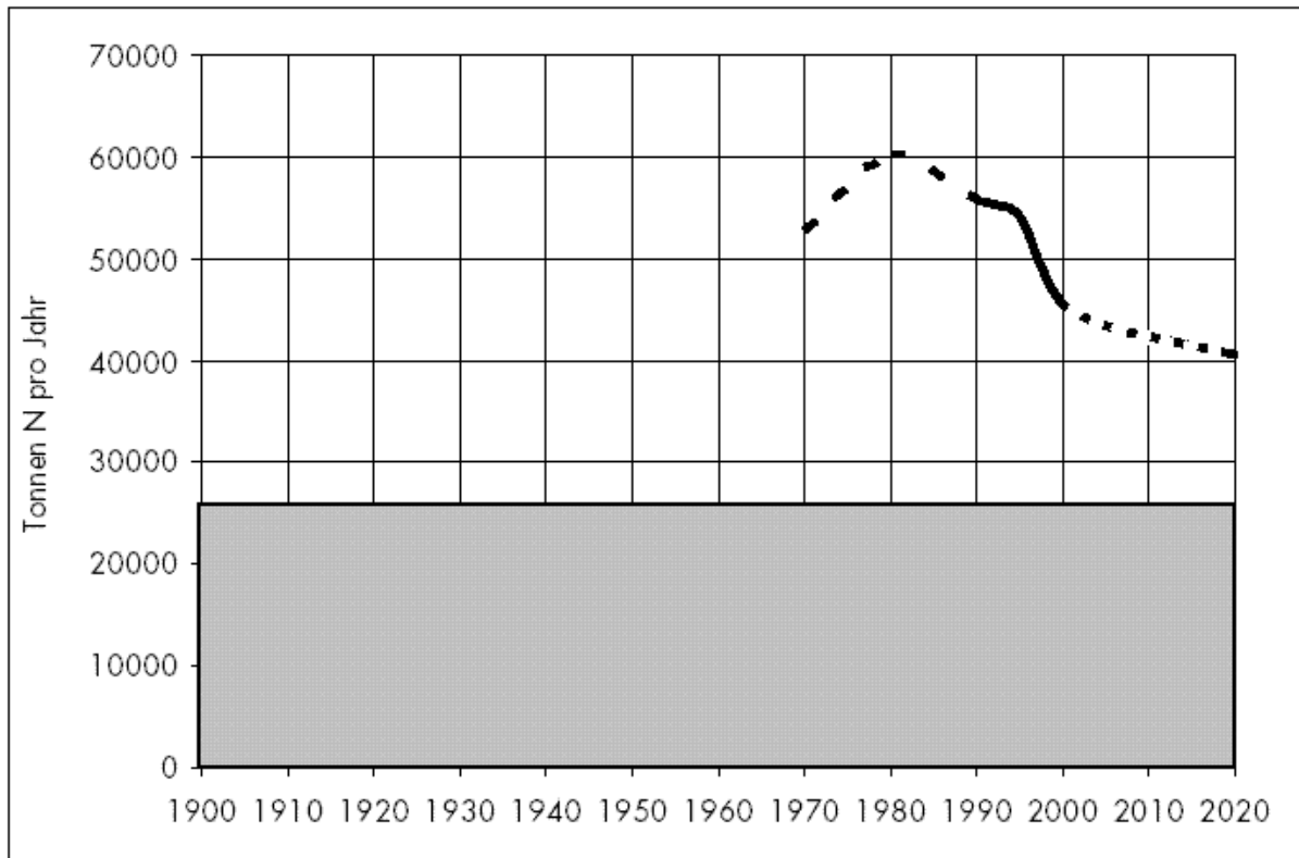
Abb. 23 Ammoniak, \text{NH}_3 Emissionsentwicklung seit 1970 und voraussichtliche Emissionen bis 2020 unter Berücksichtigung aller rechtskräftig beschlossenen Massnahmen. Grau schattiert: 'Ökologisches Ziel' Quelle: 'Weiterentwicklung des Luftreinhaltekonzeptes' Schriftenreihe Umwelt Nr. 379, BUWAL, 2005 [44]
