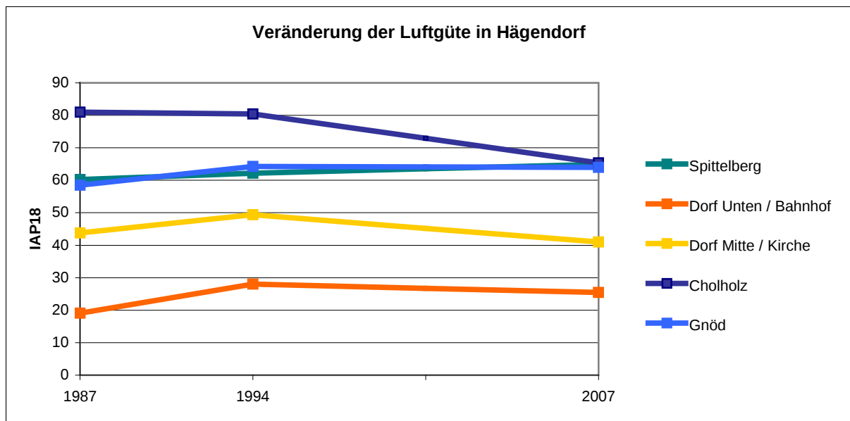
Abb. 13 Veränderung der Luftgüte an den fünf Standorten in Hägendorf 1987, 1994, 2007 Interpretationshilfe: Je höher der IAP18, desto besser die Luftqualität
