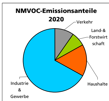
Abb. 19 Anteile der NM VOC-Emissionen im Jahre 2020 Quelle: 'Weiterentwicklung des Luftreinhaltekonzeptes' Schriftenreihe Umwelt Nr. 379, BUWAL, 2005 [44]
