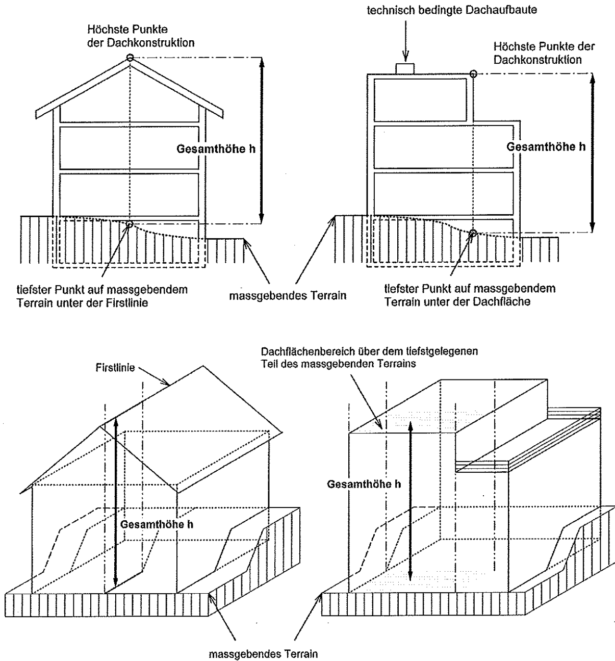
Figur 5.1 Gesamthöhe
