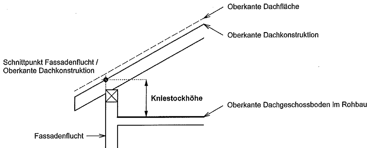
Figur 5.3 Kniestockhöhe
