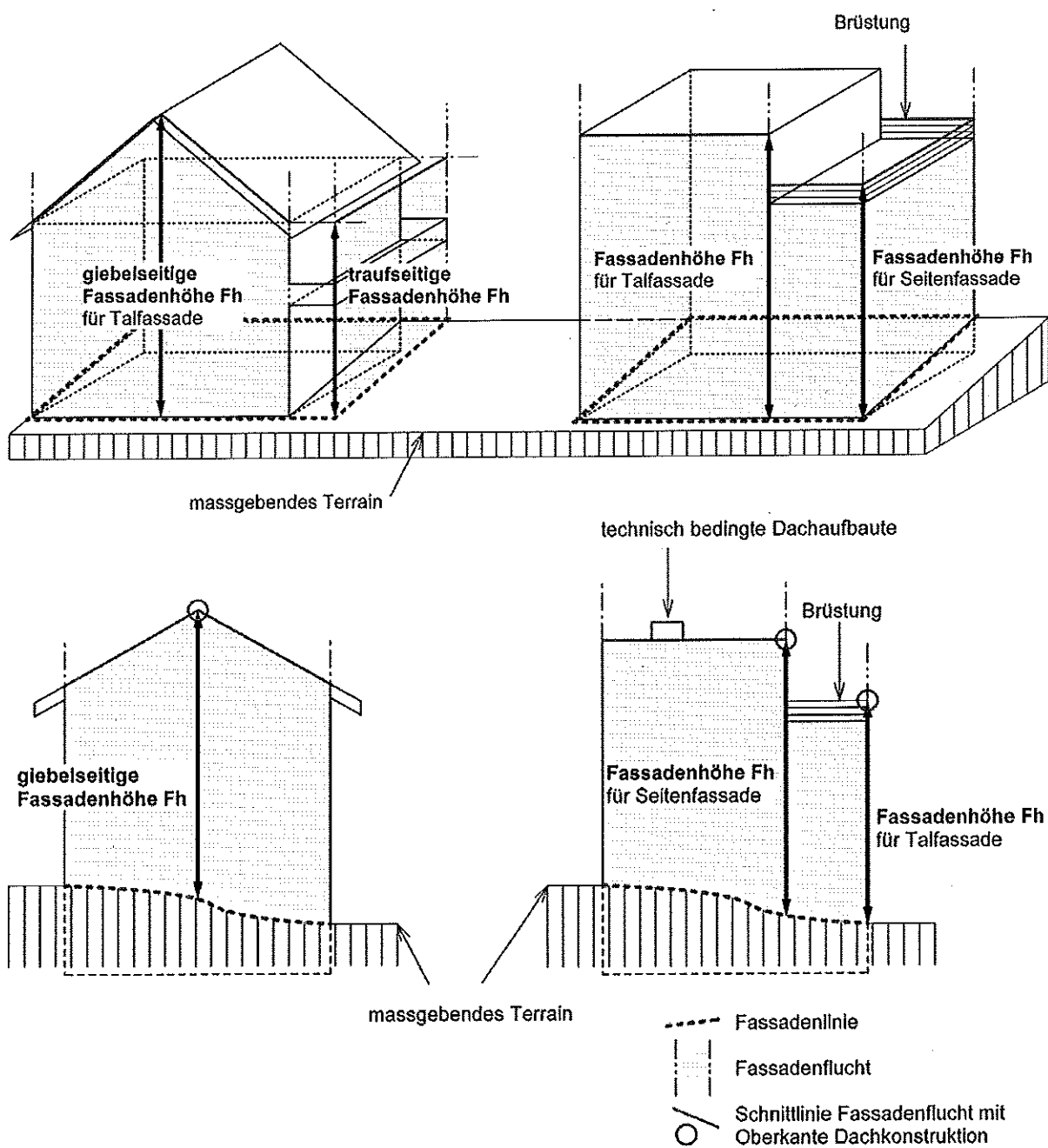
Figur 5.2 Fassadenhöhe
