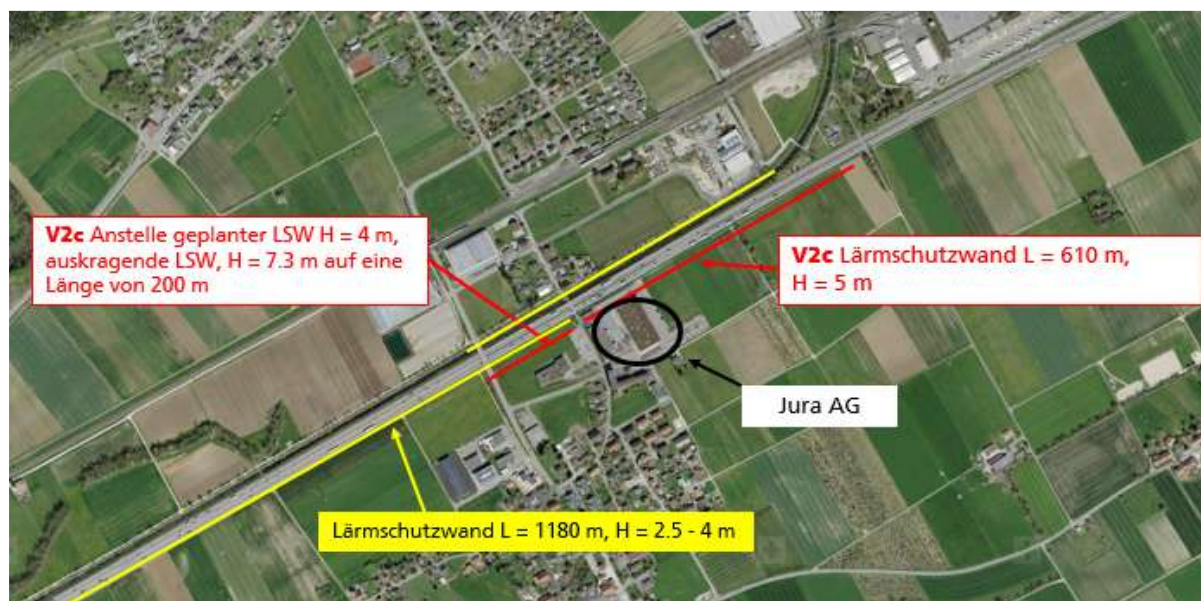
Abbildung 10: Neubau Lärmschutzwand mit Auskrugung in Niederbuchsiten (V2c)
